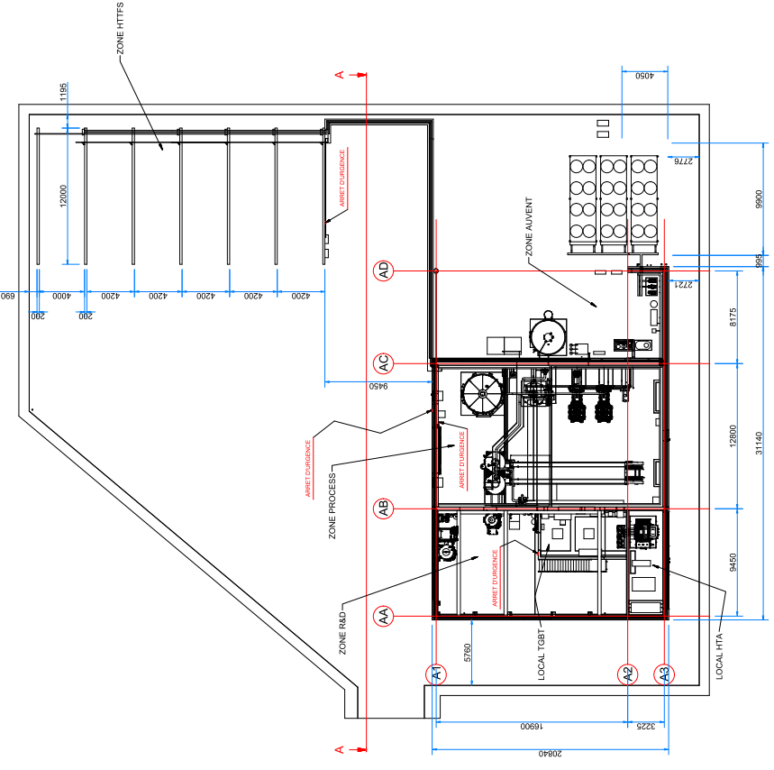
SITE DE BOUIN - VUE EN PLAN ( 1 : 150 )
